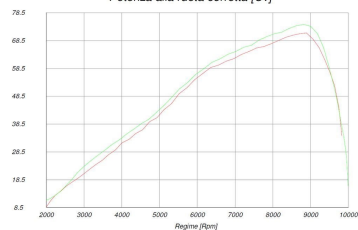
Potenza alla ruota corretta [Cv]
