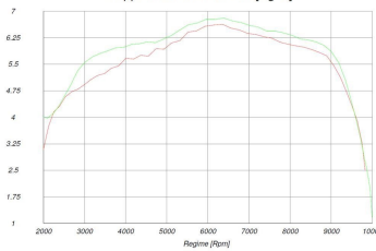
Coppia alla ruota corretta [Kg.m]
